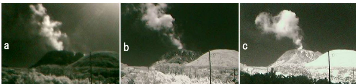
図6. 硫黄岳噴煙の近赤外面像(2006年8月8日). (a) 9:00, (b) 12:30, (c) 17:00.
