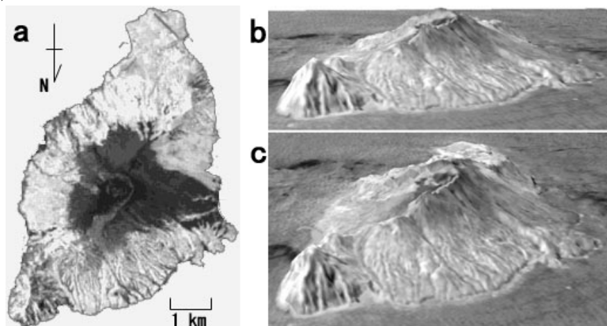
図4. 諏訪之瀬島のLANDSAT近赤外画像(a)と北方上空から見たそのSiPSEによる立体表示(b, c)。北端の侵食の進んだ山体は富立岳(536m)。
