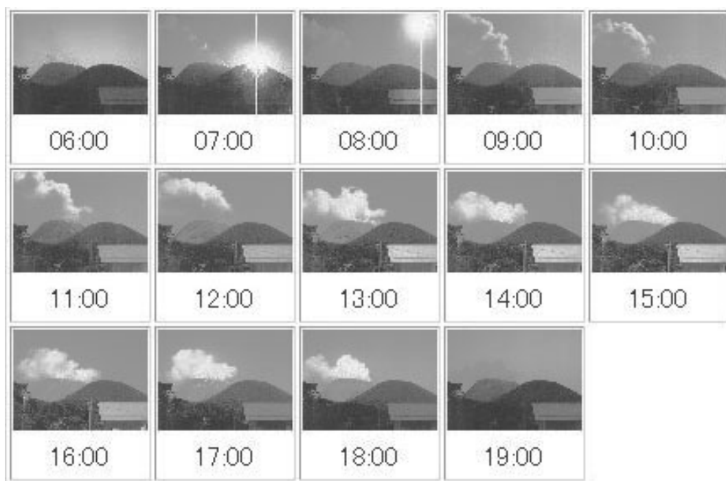
図3. 硫黄岳噴煙の1時間毎の例. 2002年8月22日.
